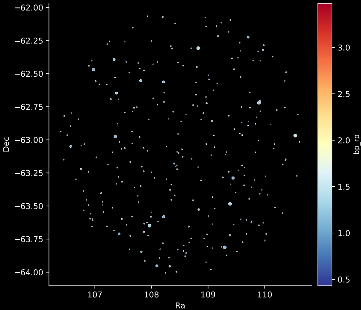
GALAH DR4 Field: [6928] Stars: 271
