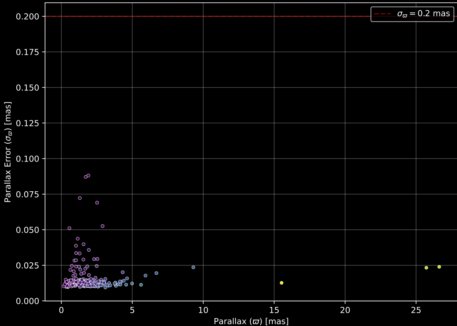
GALAH DR4 Field: [6928] Parallax Quality (n= 271)
