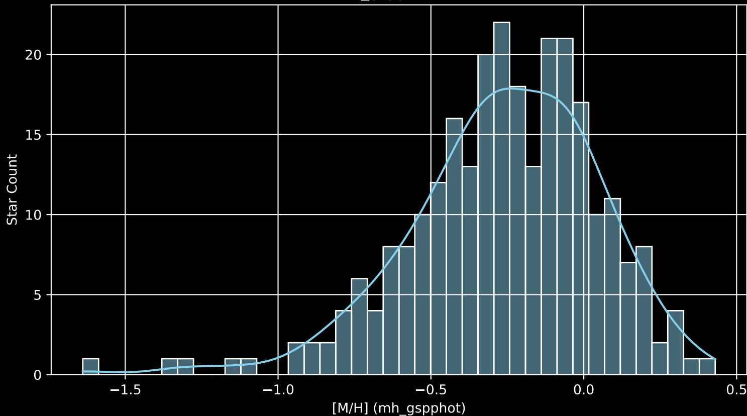
GALAH DR4 Field: [6928] [M/H] (mh_gspphot) (n= 268)
