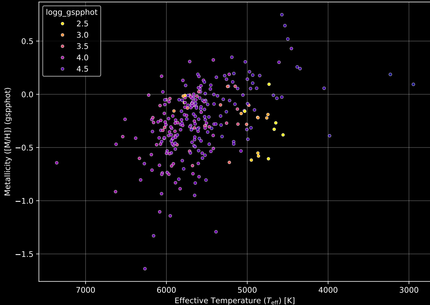
GALAH DR4 Field: [6928] Stellar Population Parameters (n= 271)
