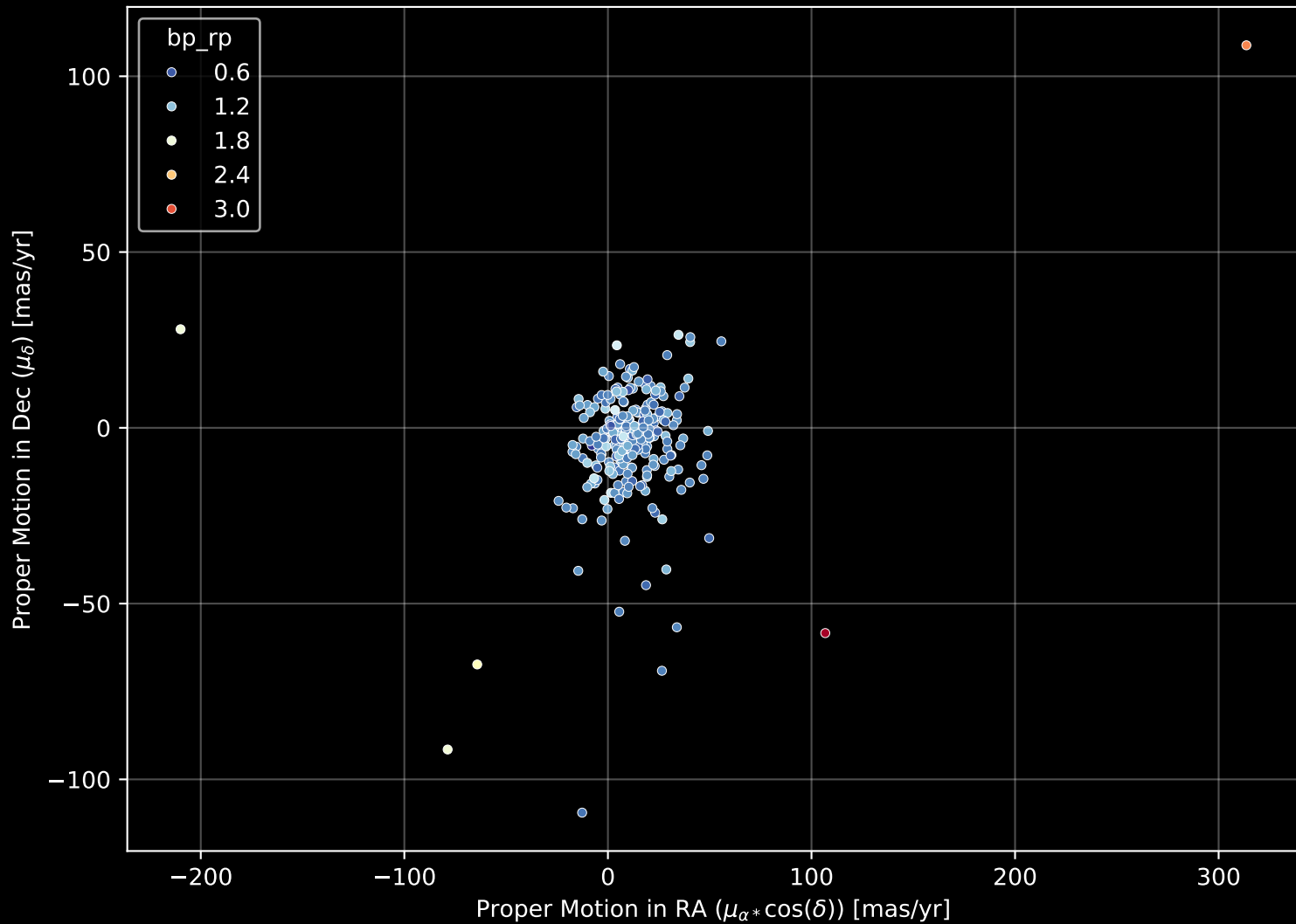
GALAH DR4 Field: [6928] Proper Motion Diagram (n= 271)
